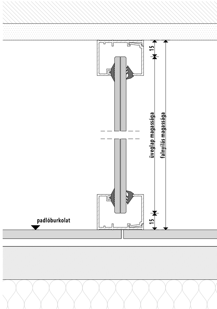
A-A metszet
